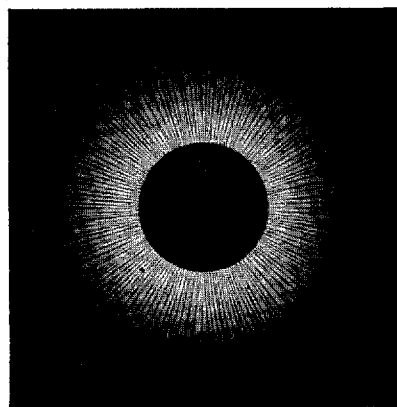
Fig. 27. Negative Figure. ( N_2 ; p = 760 ; D = 17.5 ; d_0 = 1.4 ; m = 1 ).
