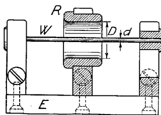
Fig. 6. Gnistbane med cylindriske Elektroder, nemlig Traaden W og Ringen R . E er en Ebonitplade
