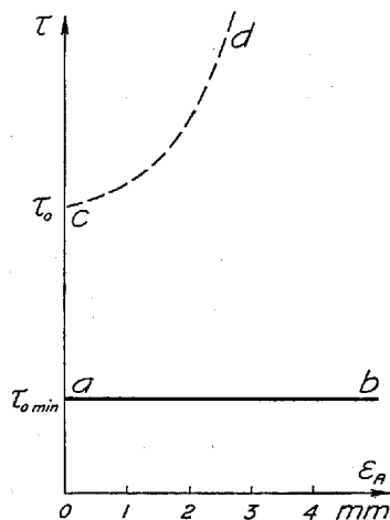
Fig. 2. Skematisk Fremstilling af Forsinkelsens Afhængighed af Anodens Tilbagetrækning \varepsilon_A . Kurve ab gælder for ren Katode i Normalstilling ( \varepsilon_c = 0 ) ( l = 20 mm). Kurve cd for Katode enten fedtet eller stærkt tilbagetrukket eller begge Dele.
