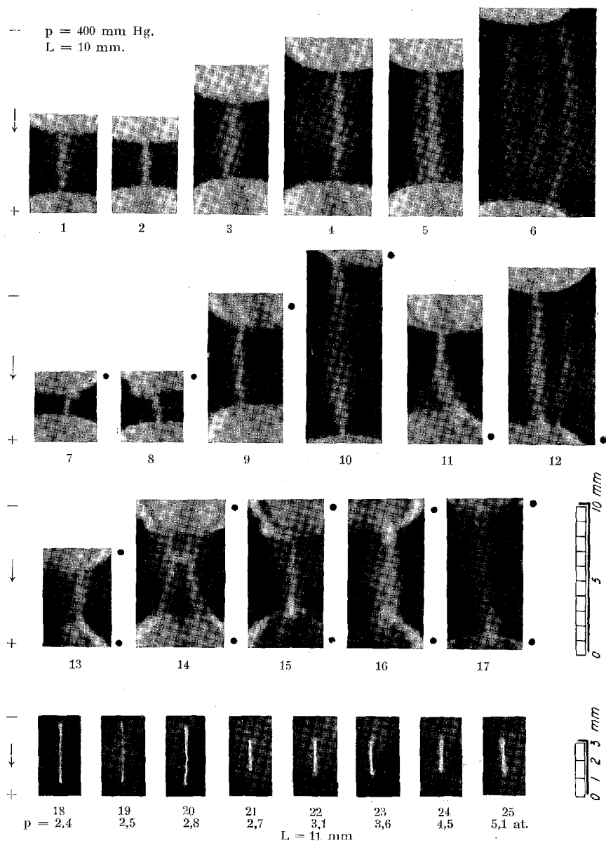
Gnister i atmosfærisk Luft. Nr. 1—17 ved et Tryk af p=400 \text{ mm Hg.} Nr. 18—25 ved Tryk fra 2,4 til 5,1 at. I Nr. 1—6 og 18—25 er Elektroderne rene. I de øvrige angiver en sort Prik tilhøjre for Billedet af en Elektrode, at denne er forurenet ved en tynd Oliehinde.
