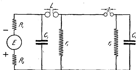
Fig. 7. Skematisk Diagram af den ved Optagelsen af Billederne paa Plan I-VI og VI-VII benyttede Forsøgsopstilling. R_1 , R_2 , r_1 og r_2 meget store Modstande paa flere Megohm (Grifler). C_1 's Kapacitet ca. 2000 cm; C_2 's som Regel kun nogle faa cm.
