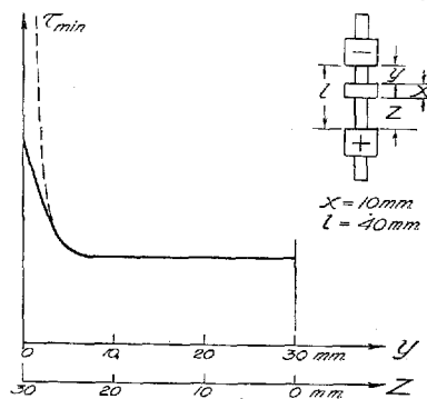
Fig. 5. Gnistforsinkelsens Afhængighed af Ringens Stilling. Den fuldt optrukne Kurve gælder for ren Anode, den punkterede for fedtet Anode
